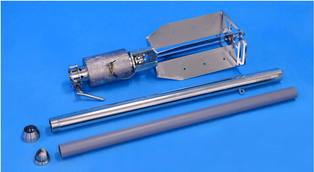
采样器示意图 13.570
