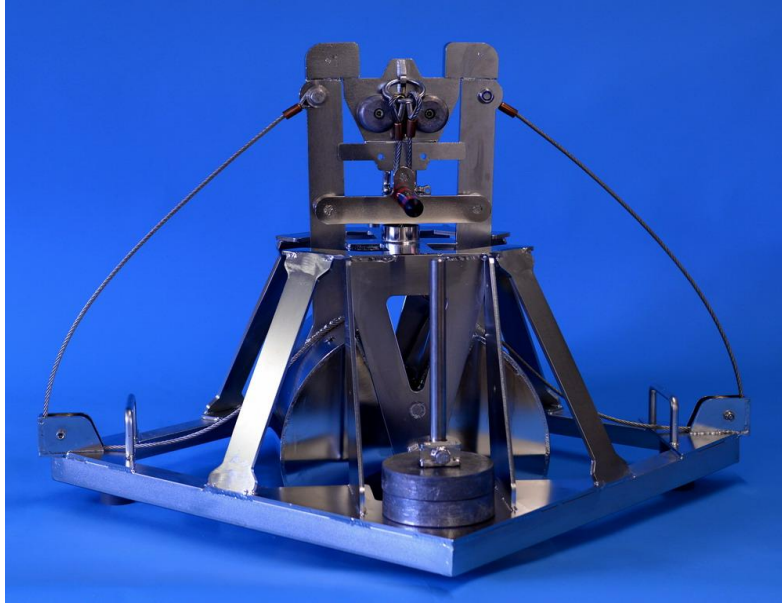
Day 静力采泥器
